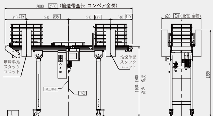
*外形尺寸圖为A-40基本尺寸。□内表示A-70的尺寸。 圖面はA-40です。□は、A-70の寸法を示します。 This drawing is for A-40. Figures in □ show the sizes of A-70 II.
